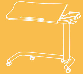
MO-4813-00006 TABLE À MANGER GRAND PLATEAU INCLINABLE + PETIT PLATEAU LATÉRAL AVEC GALERIE PIÈTEMENT C - CHANTS ABS HAUTEUR VARIABLE DIM : L95 X H75/109 X P45 CM
